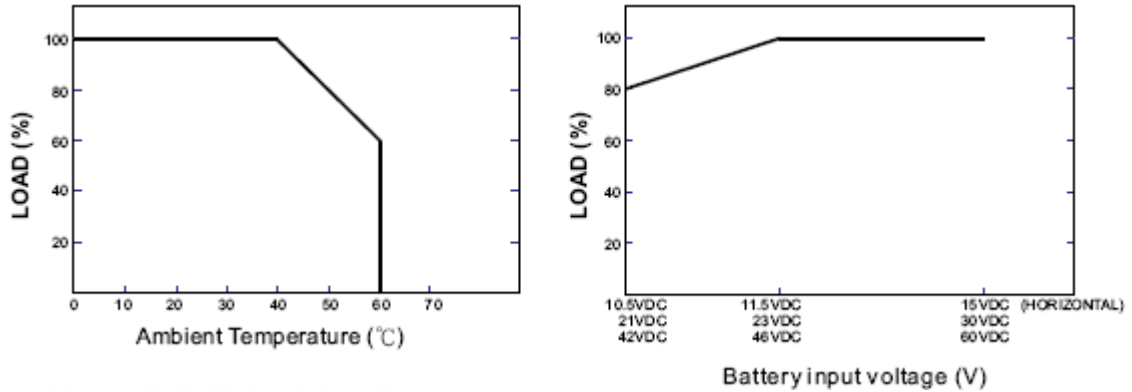
Figura 12 - Curvas de Deriva
