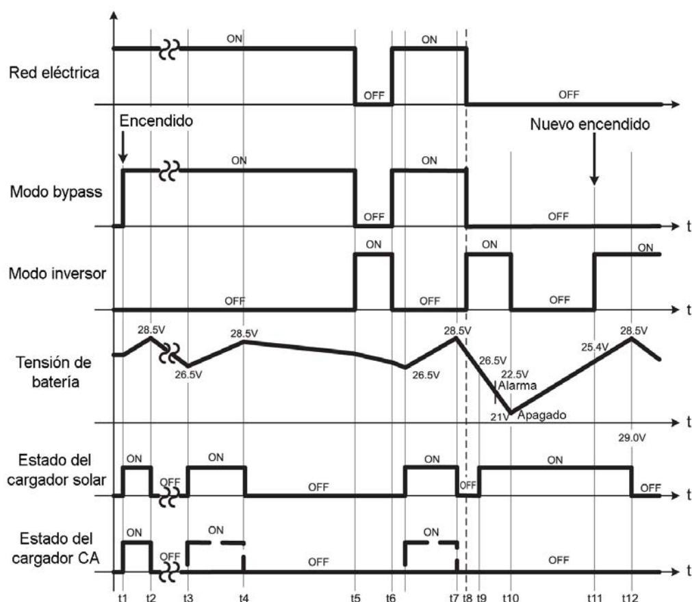
Figura 5 - Explicación del Modo Funcionamiento SAI
