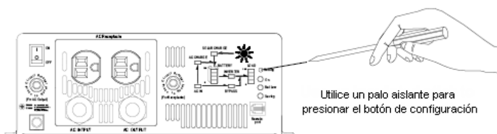
Figura 7 – Ajuste del modo de salida, tensión de salida, frecuencia y modo ahorro de energía
